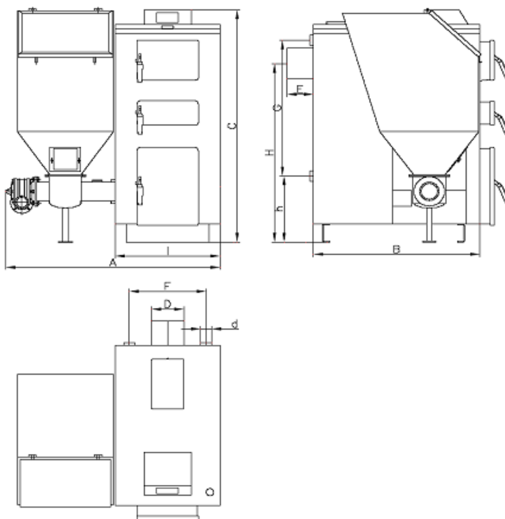
SCHEMAT KOTŁA UNI PLUS 15-50 KW
